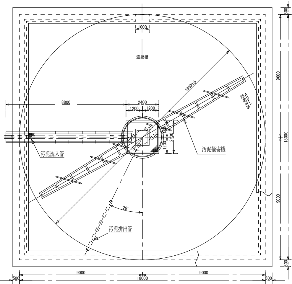
濃縮槽 平面図
