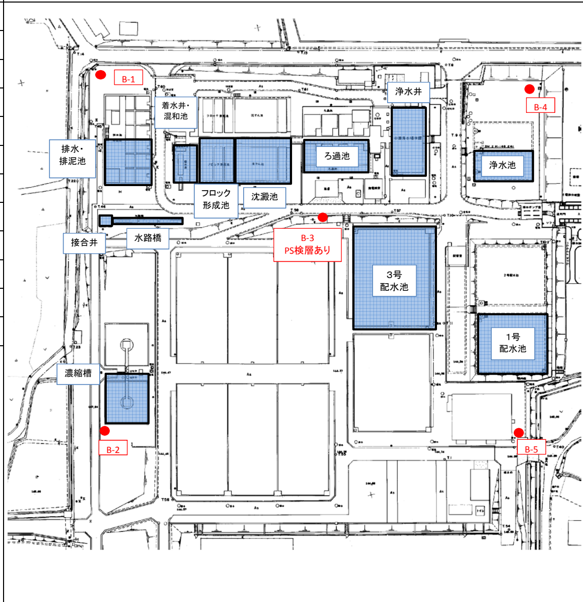
位置図
